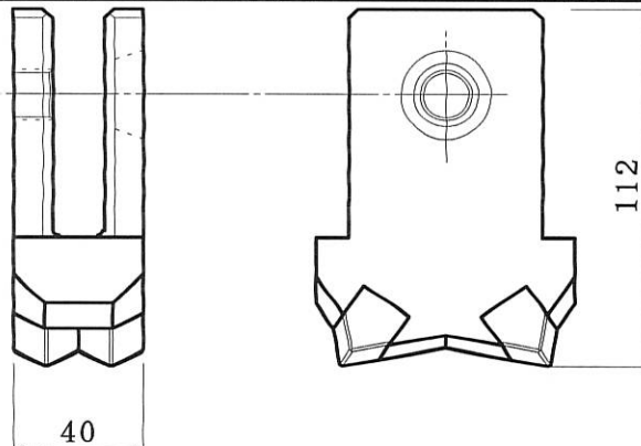
右センター刃
