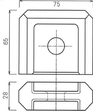
2 27.5巾ケーシングビット
