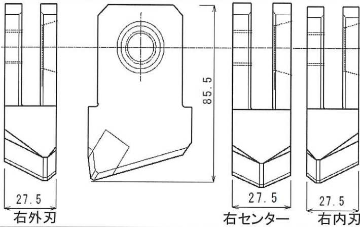
3 27.5巾ケーシングビット 両刃
