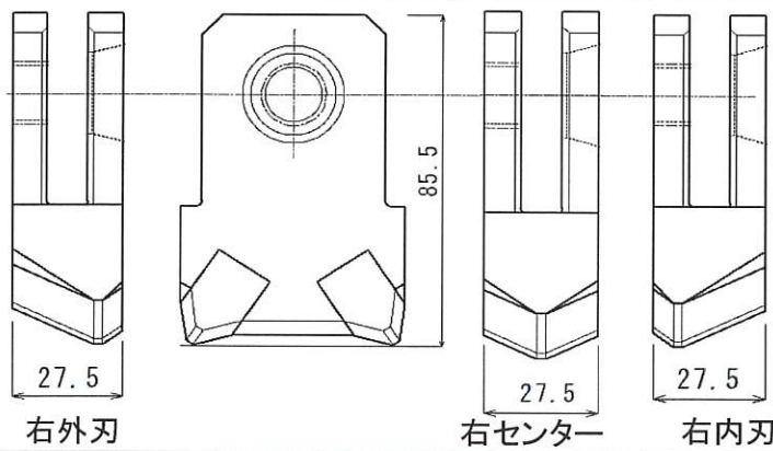
4 40巾ケーシングビット アゴ上100
