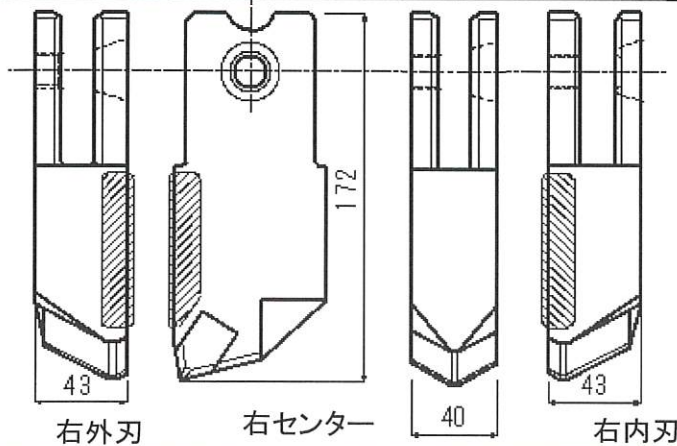
4 40巾ケーシングビット アゴ上100
